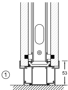
Modulo vidrio continuo doble Continuous double pane glass module Module avec double vitrage continu Durchgehendes Doppelglasmodul
