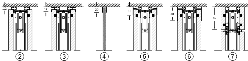
Opciones zócalo superior Upper skirting options Options socle supérieur Optionen Sockel oben
