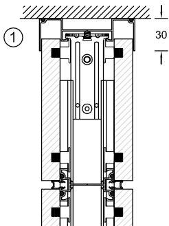
Módulo ciego Blind module Module à âme pleine Blindmodul
